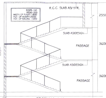
SECTION-AA' SCALE-1:200
