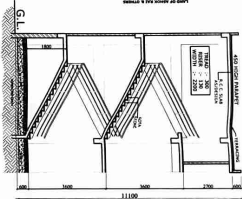
SECTION-AA SCALE-1:200
