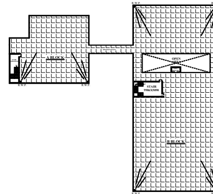
TERRACE PLAN SCALE: 1/50
