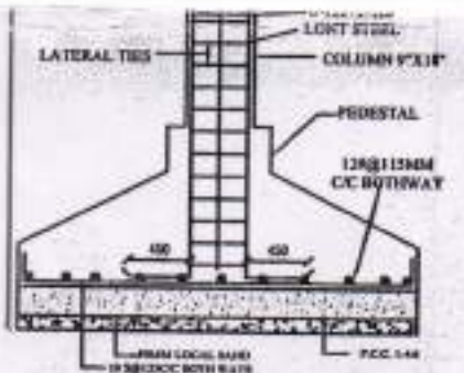
DETAIL OF COLUMN (N.T.S.)
