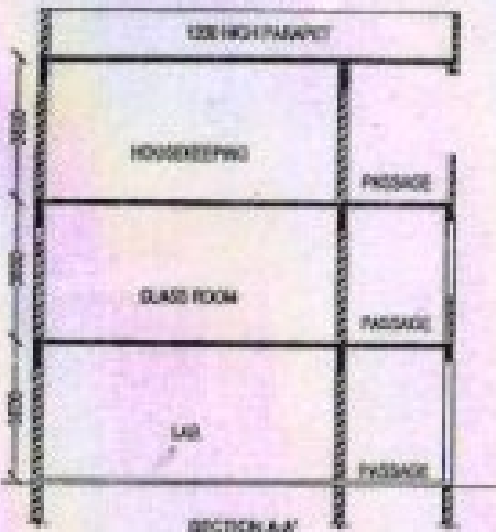
SECTION A-A SCALE: 1:50
