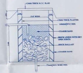
SECTION OF S.P. FOR R.W.P. (SCALE :-N.T.S.)
