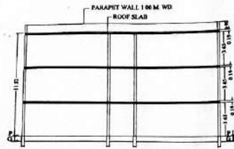
SECTION A-B
