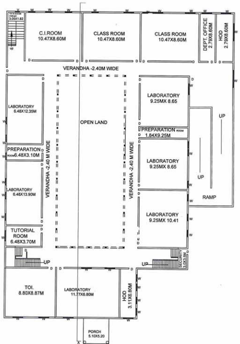
S.F.PLAN(scale 1:100)
