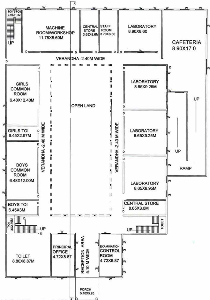
G.F. PLAN(scale 1:100)
