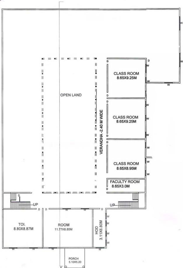
T.F.PLAN(scale 1:100)
